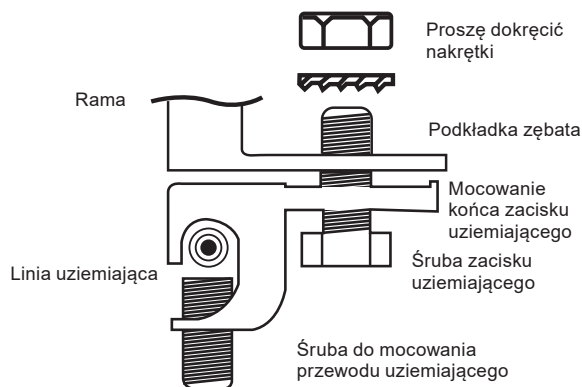
Rysunek 12 Metoda uz iemienia otworu montażowego
