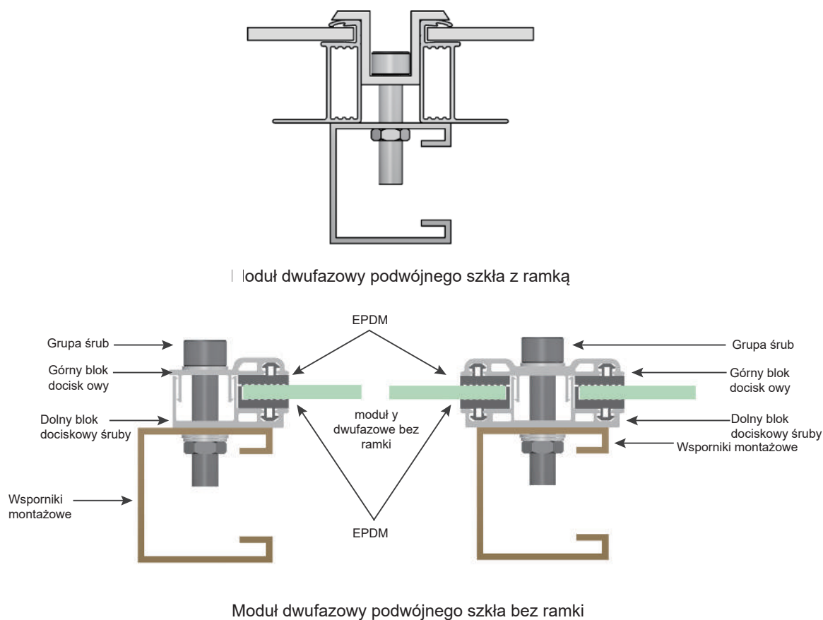
Rysunek 8 Schemat montażu zacisku modułu dwufazowego
