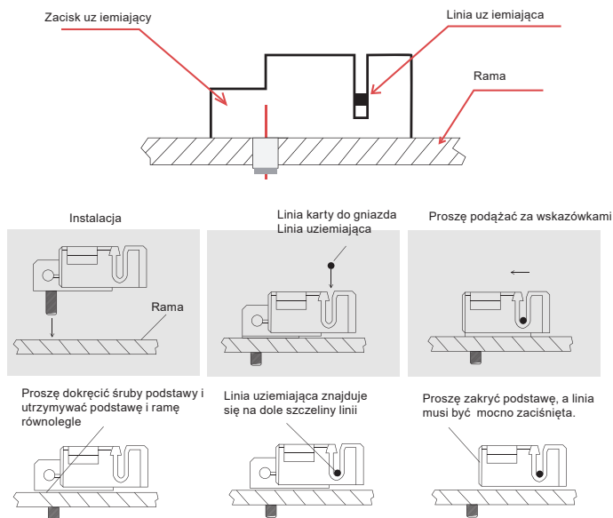
Rysunek 11 Metoda montażu zacisku uz iemającego
