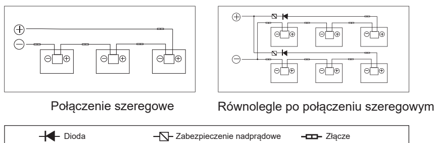
Rysunek 10 Schemat elektryczny obwodów szeregowych i równoległych
